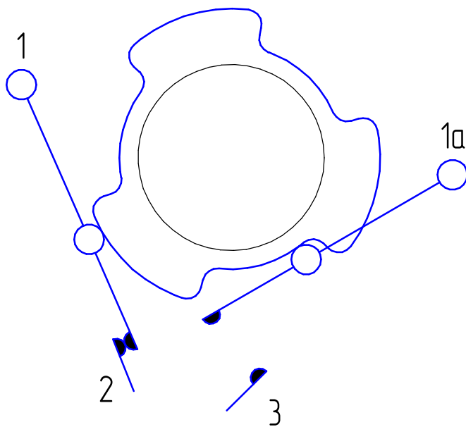
Позиция 4 Контакты 1-2 замкнуты, 1а-3 разомкнуты
