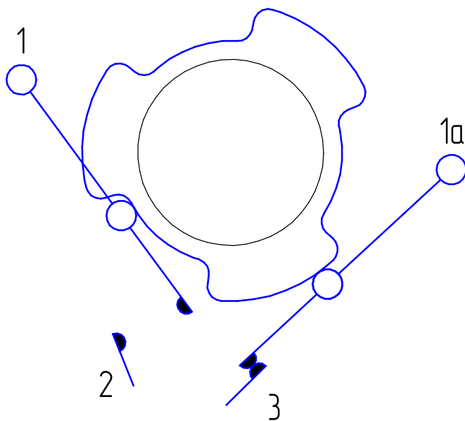
Позиция 2 Контакты 1-2 разомкнуты, 1а-3 замкнуты
