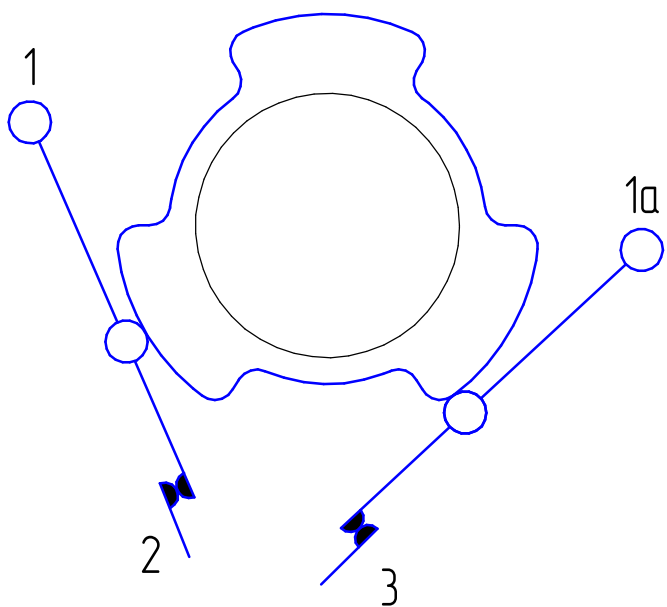
Позиция 1 Контакты 1-2 и 1а-3 замкнуты
