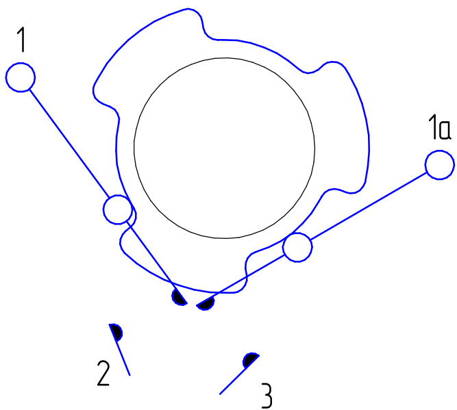
Позиция 3 Контакты 1-2 и 1а-3 разомкнуты
