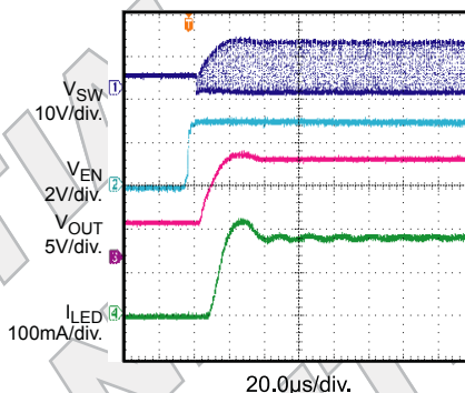
Enable Startup
