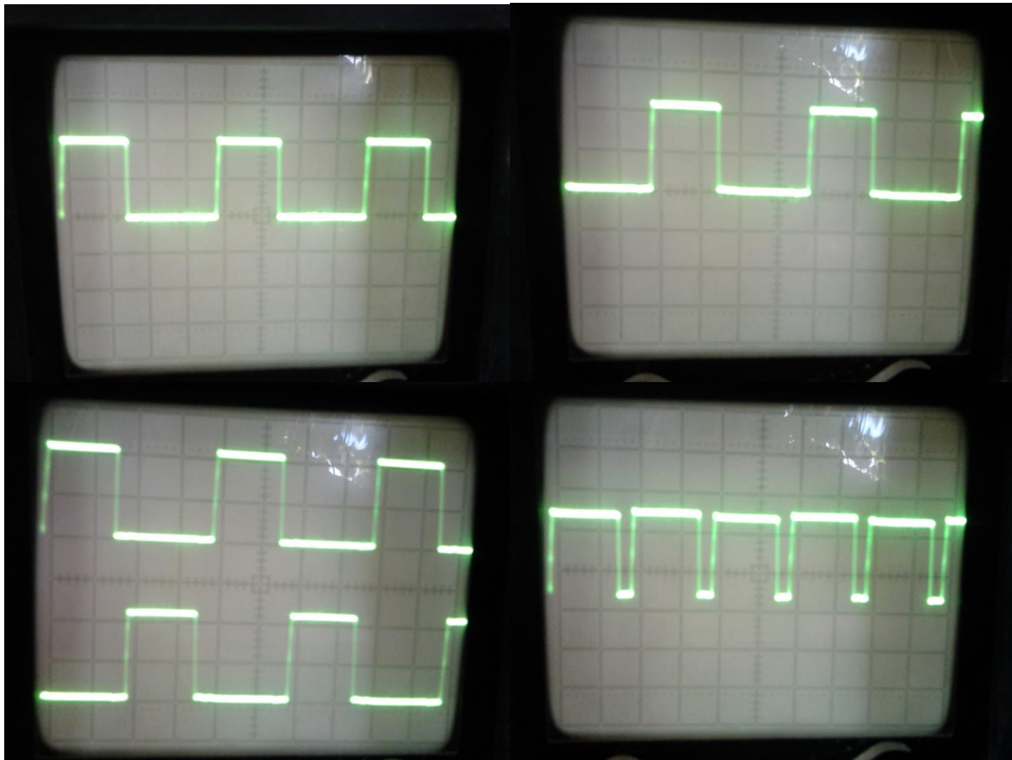
Выход с TL 494 (5 вольт\ 1 мкс)
