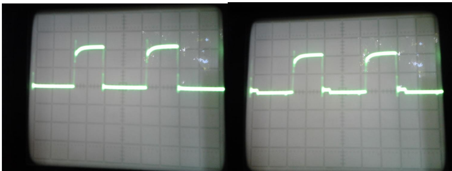
Выход с IR 2110 (5 вольт\ 1 мкс)
