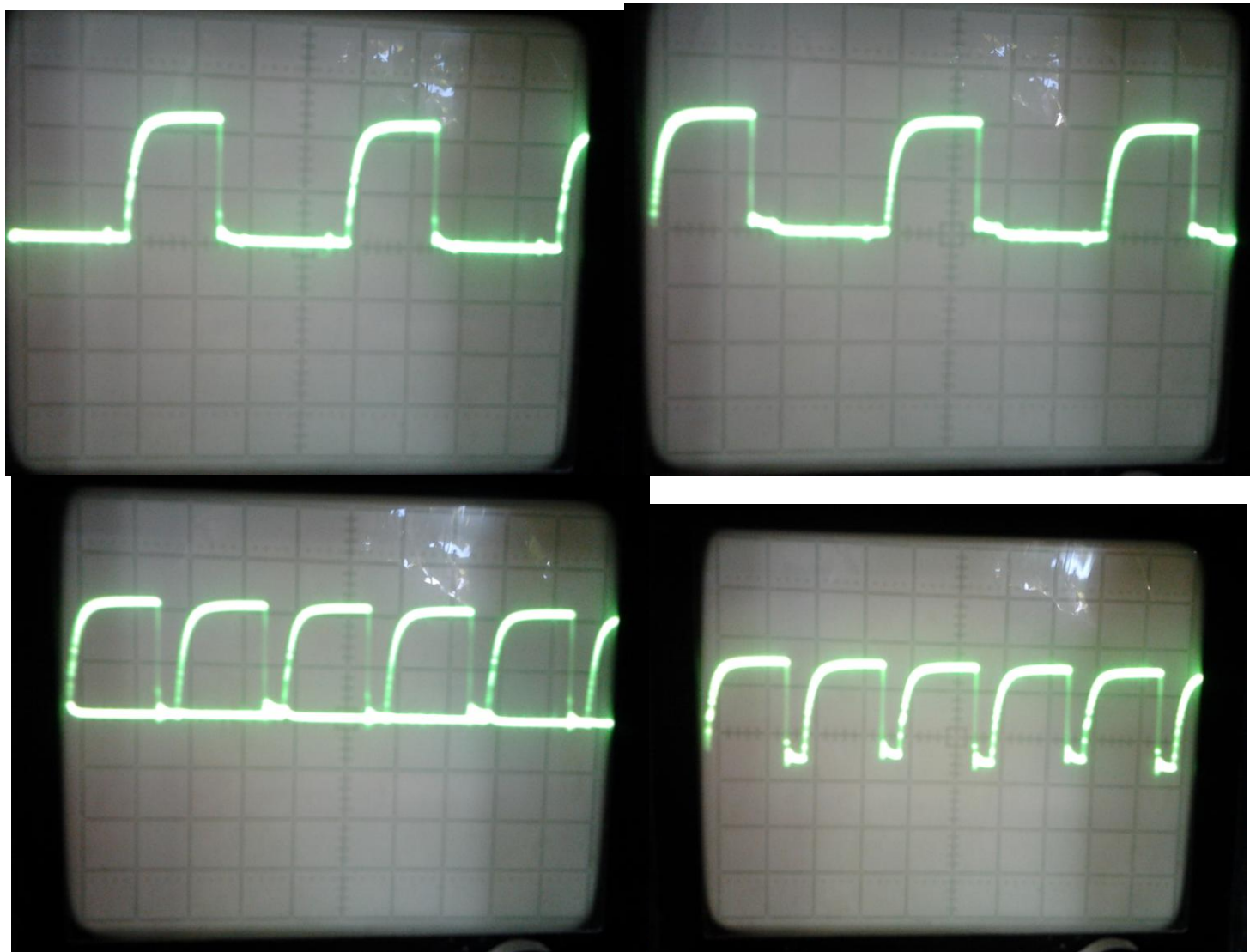
На затворах транзисторов (5 вольт\ 1 мкс)
