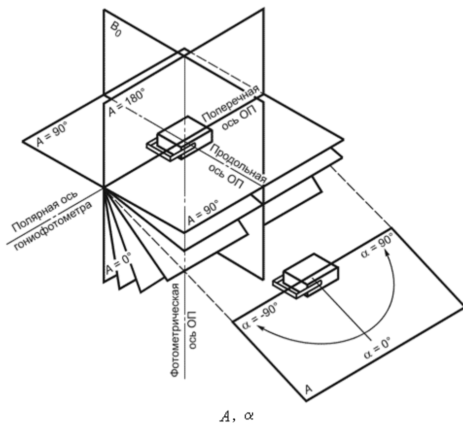
Рисунок Б.1 - Системы фотометрирования
