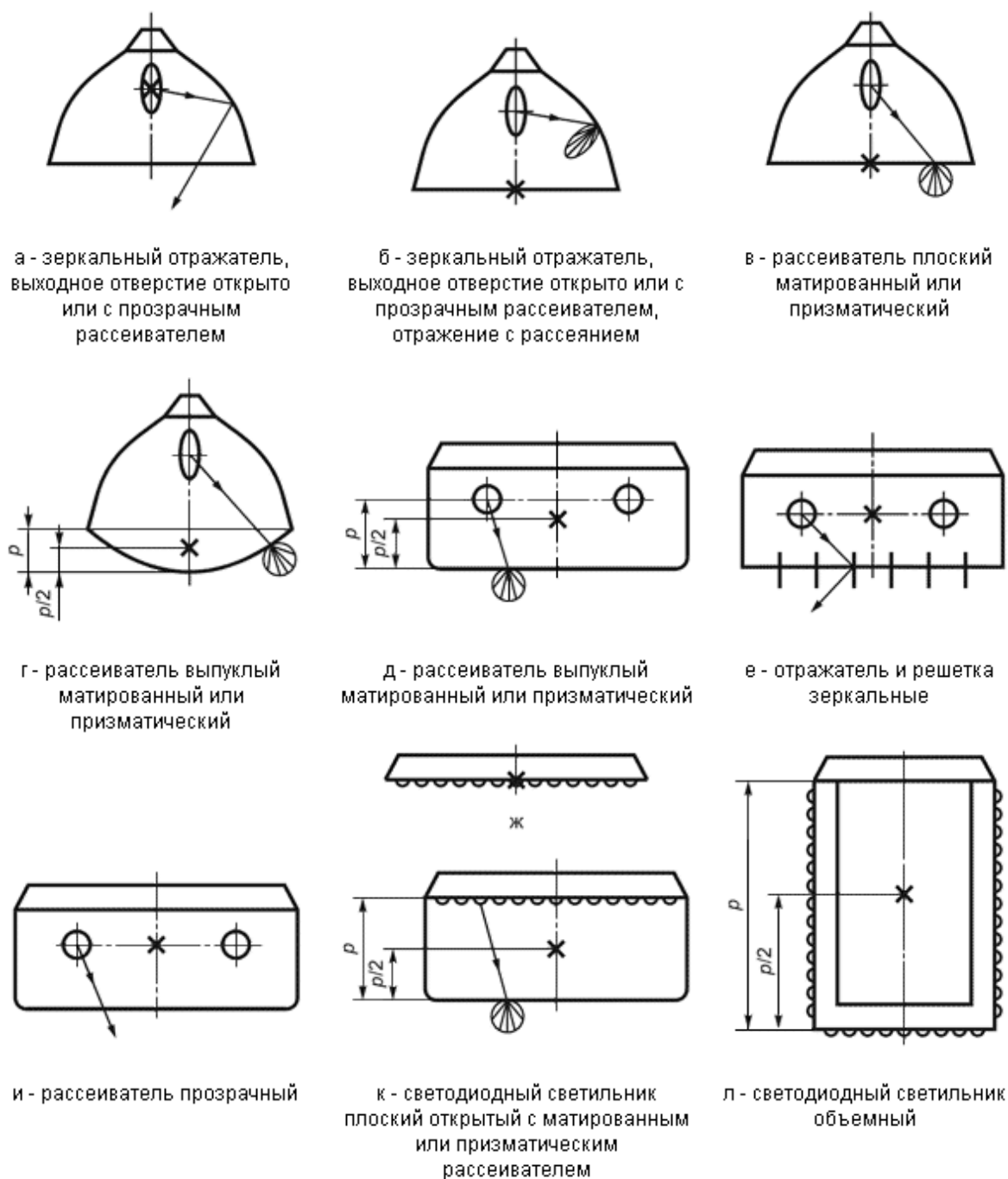
Рисунок В.1 - Положение фотометрического центра осветительного прибора
