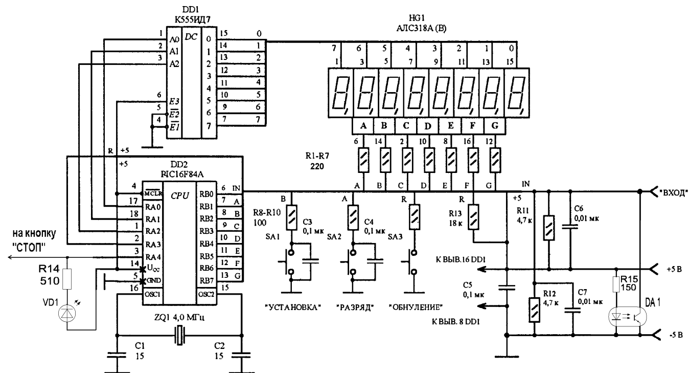
Рис. 37. Счетчик витков
