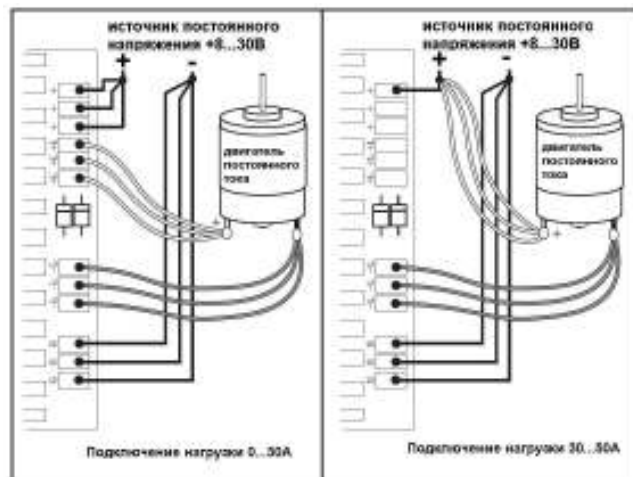
Рис.3. Схема подключений
