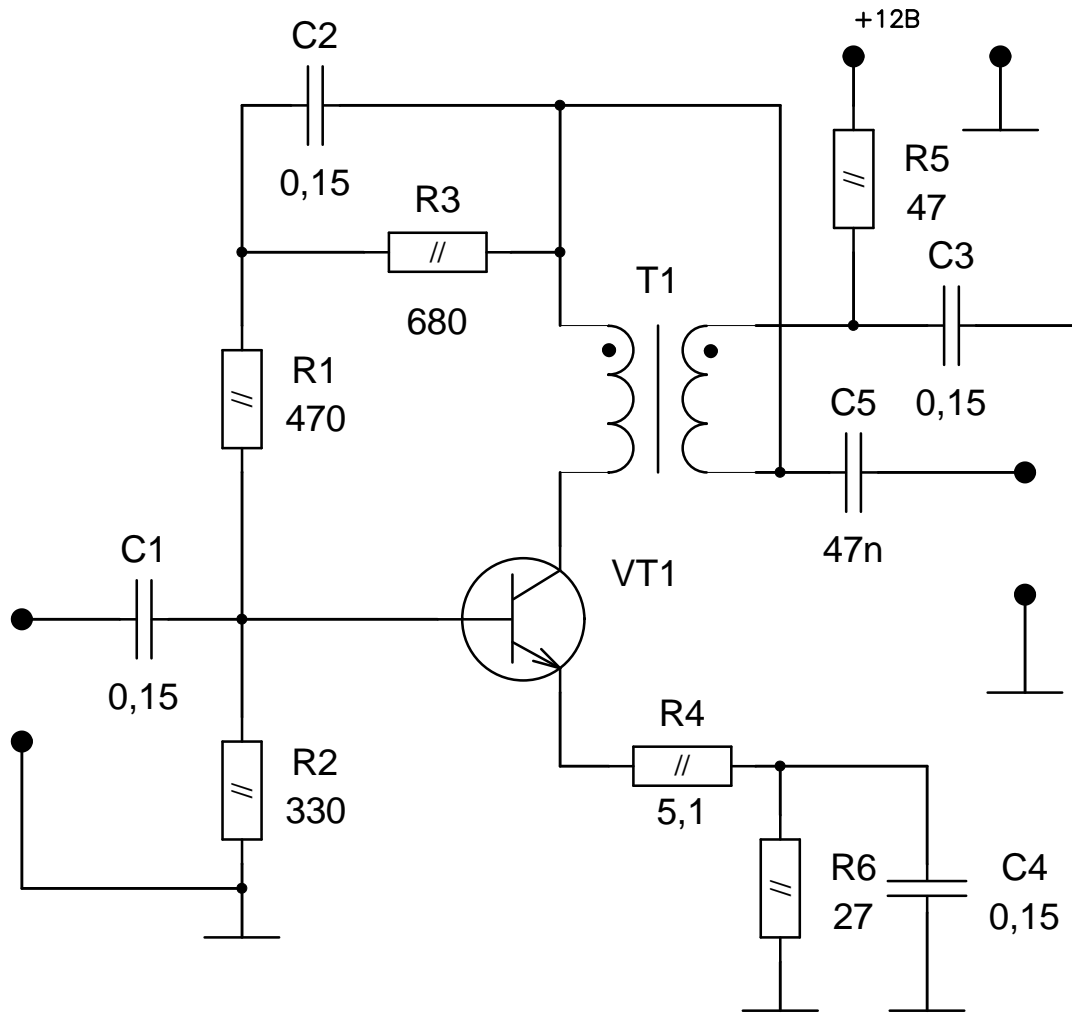
Пример широкополосного усилителя
