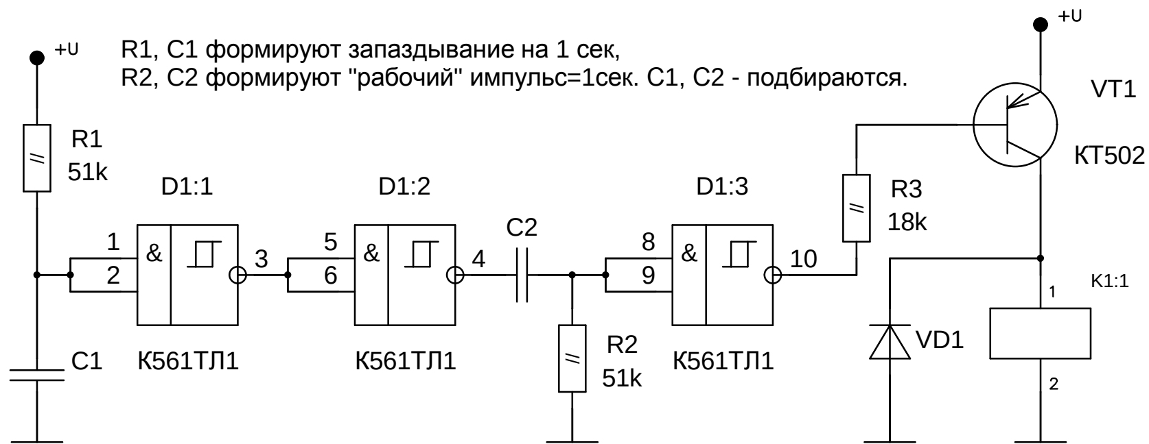
Схема запаздывания
