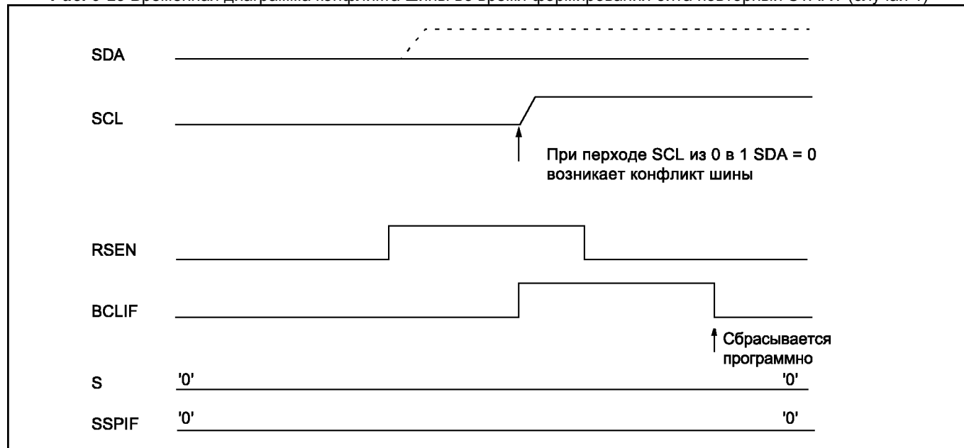
Рис. 9-23 Временная диаграмма конфликта шины во время формирования бита повторный START (случай 1)
