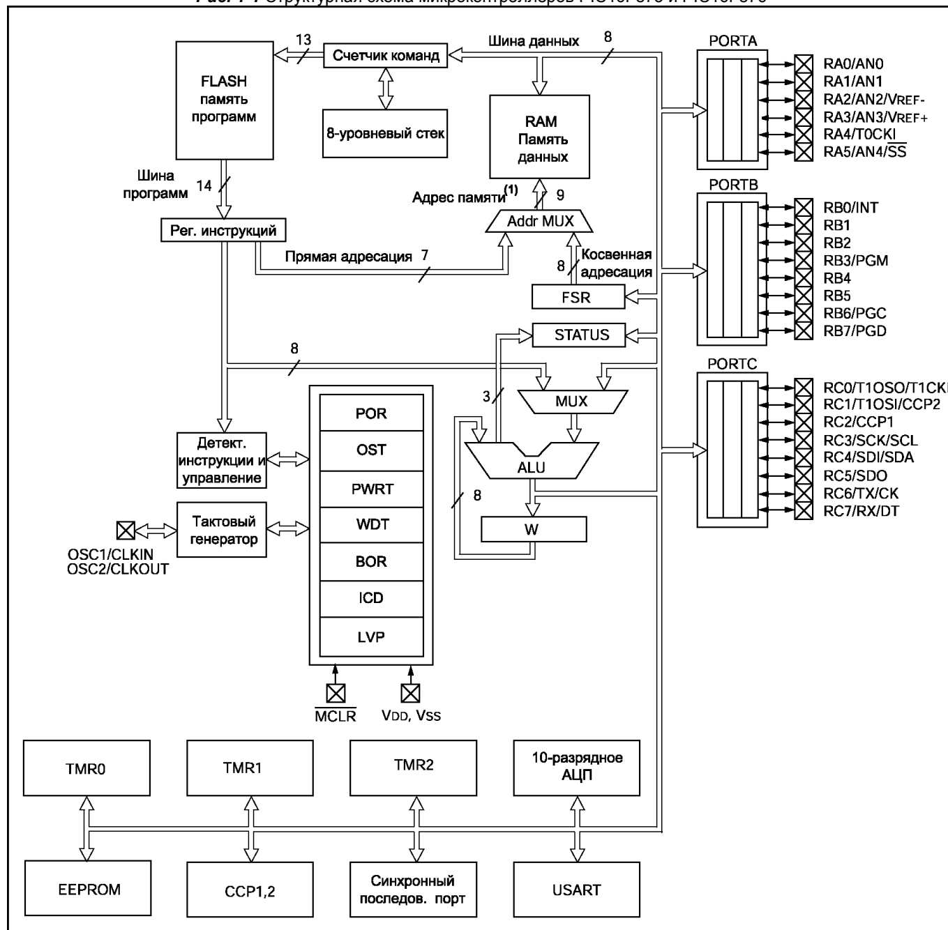
Рис. 1-1 Структурная схема микроконтроллеров PIC16F873 и PIC16F876
