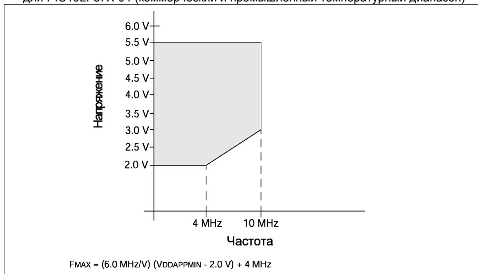
Рис. 15-2 График рекомендованных комбинаций значений напряжения питания и тактовой частоты для PIC16F87X-04 (коммерческий и промышленный температурный диапазон)
