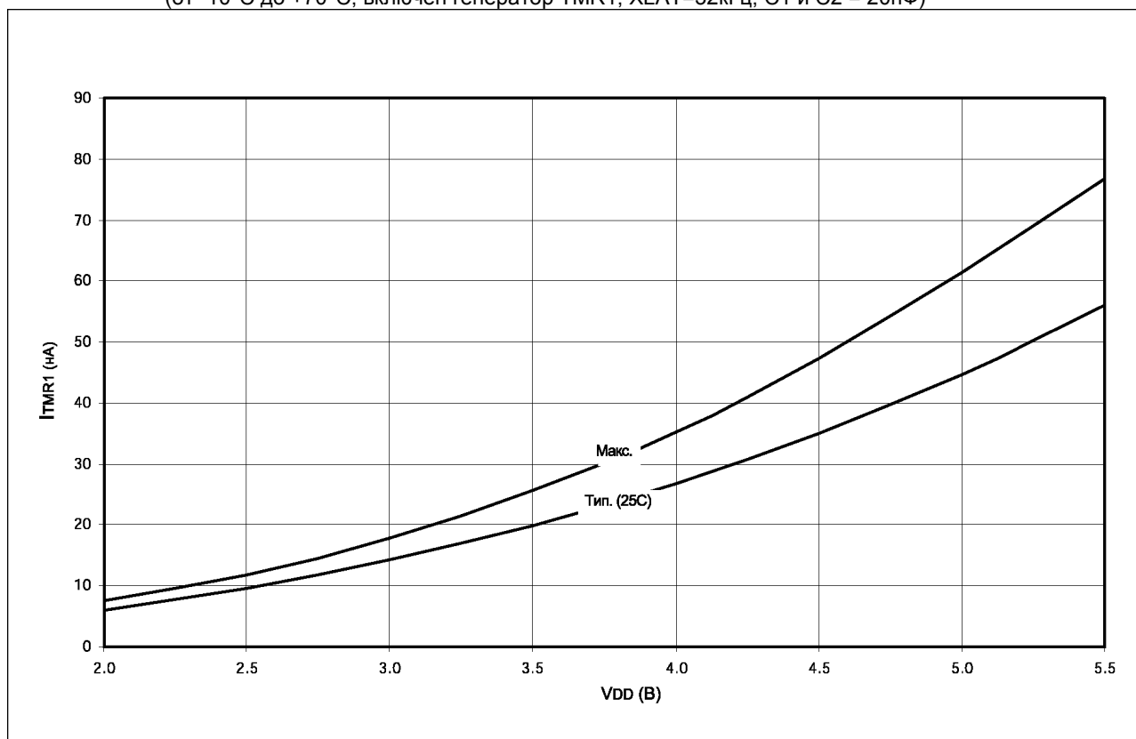
Рис. 16-12 График зависимости типового и максимального \Delta I_{TMR1} от V_{DD} при различных температурах (от -10^{\circ}\text{C} до +70^{\circ}\text{C} , включен генератор TMR1, XLAT=32кГц, C1 и C2 = 20пФ)
