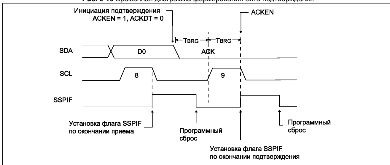
Рис. 9-16 Временная диаграмма формирования бита подтверждения
