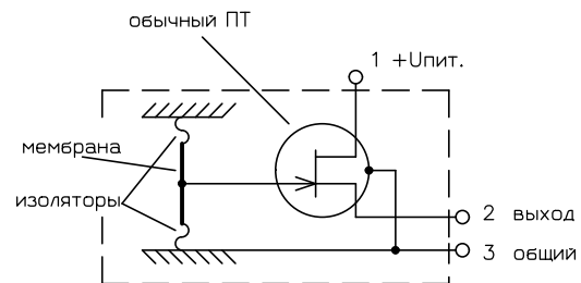
начинка электретного микрофона
