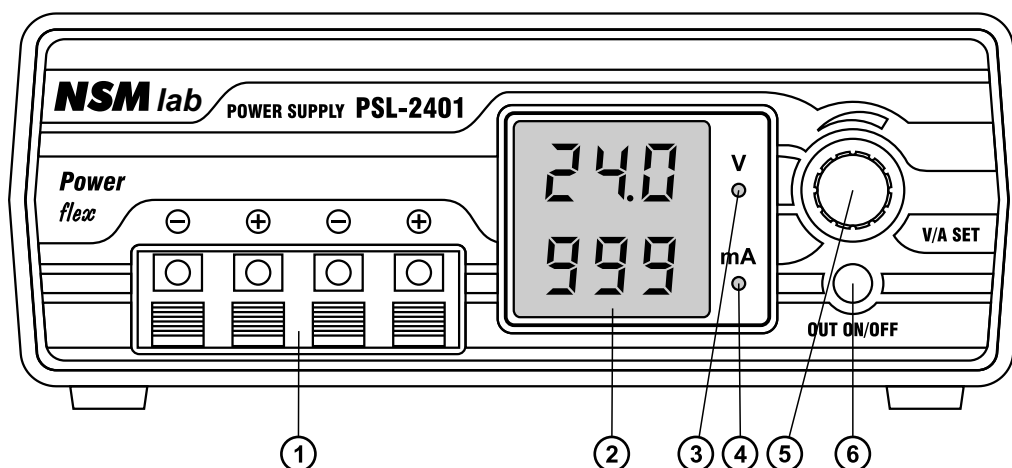
Рис. 1. Передняя панель источника.
