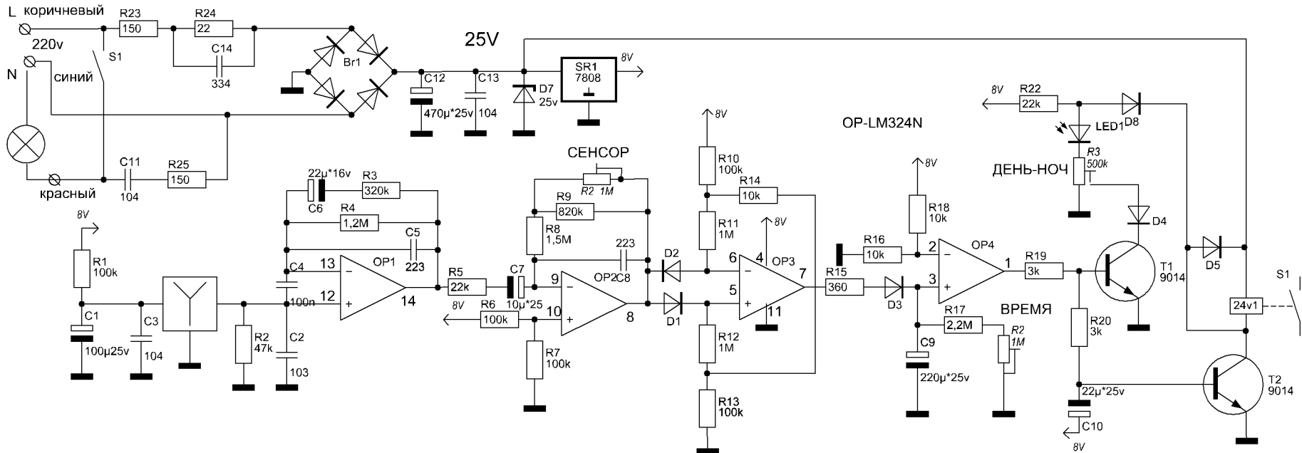
Схема китайского прожектора с датчиком движения LX-01
