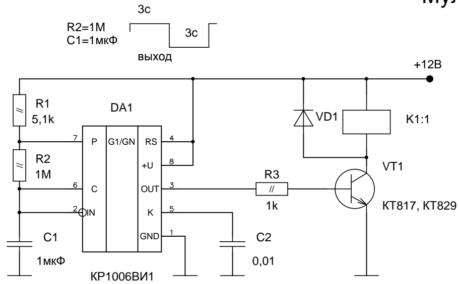
Мультивибратор на KP1006ВИ1
