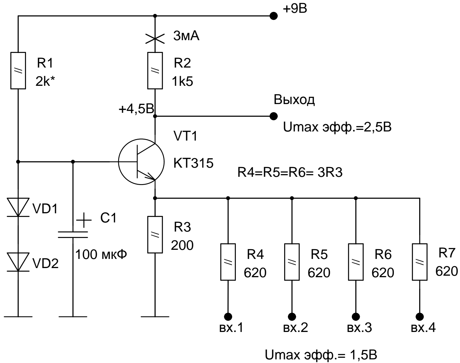
Сумматор НЧ сигнала
