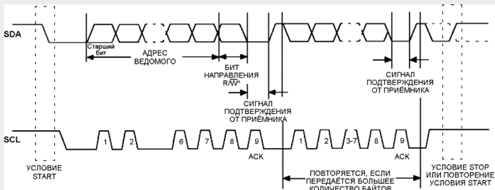
Рис. 5. Передача данных по двухпроводной последовательной шине
