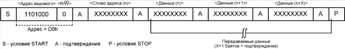
Рис. 6. Запись данных - режим ведомого приёмника
