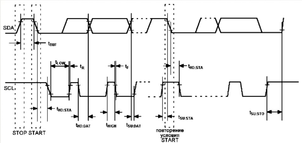
Рис. 8. Временная диаграмма
