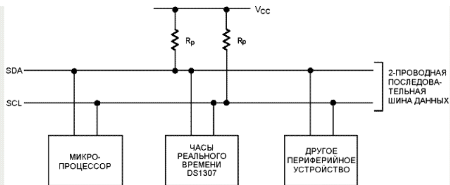
Рис. 4. Типовая конфигурация двухпроводной шины
