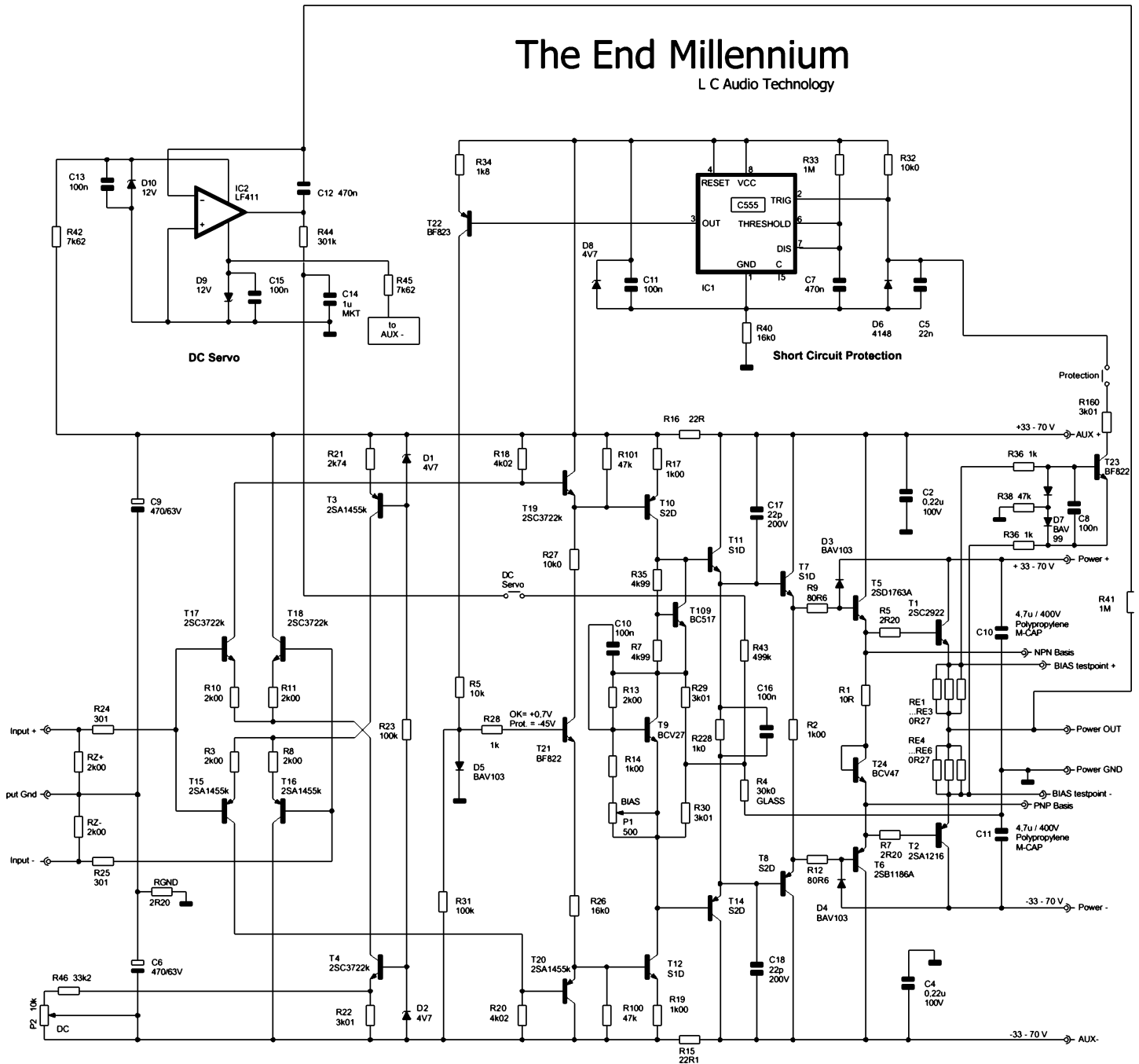
Рисунок 2.50. Схема High-End усилителя End Millennium небольшой датской фирмы LC Audio
