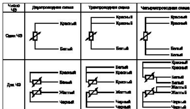
Рисунок 1 — Схемы соединения внутренних проводов
