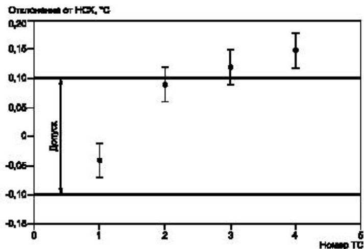
Рисунок В.1 — Условия приемки и отбраковки ТС класса АА по результатам измерений при 0 °С
