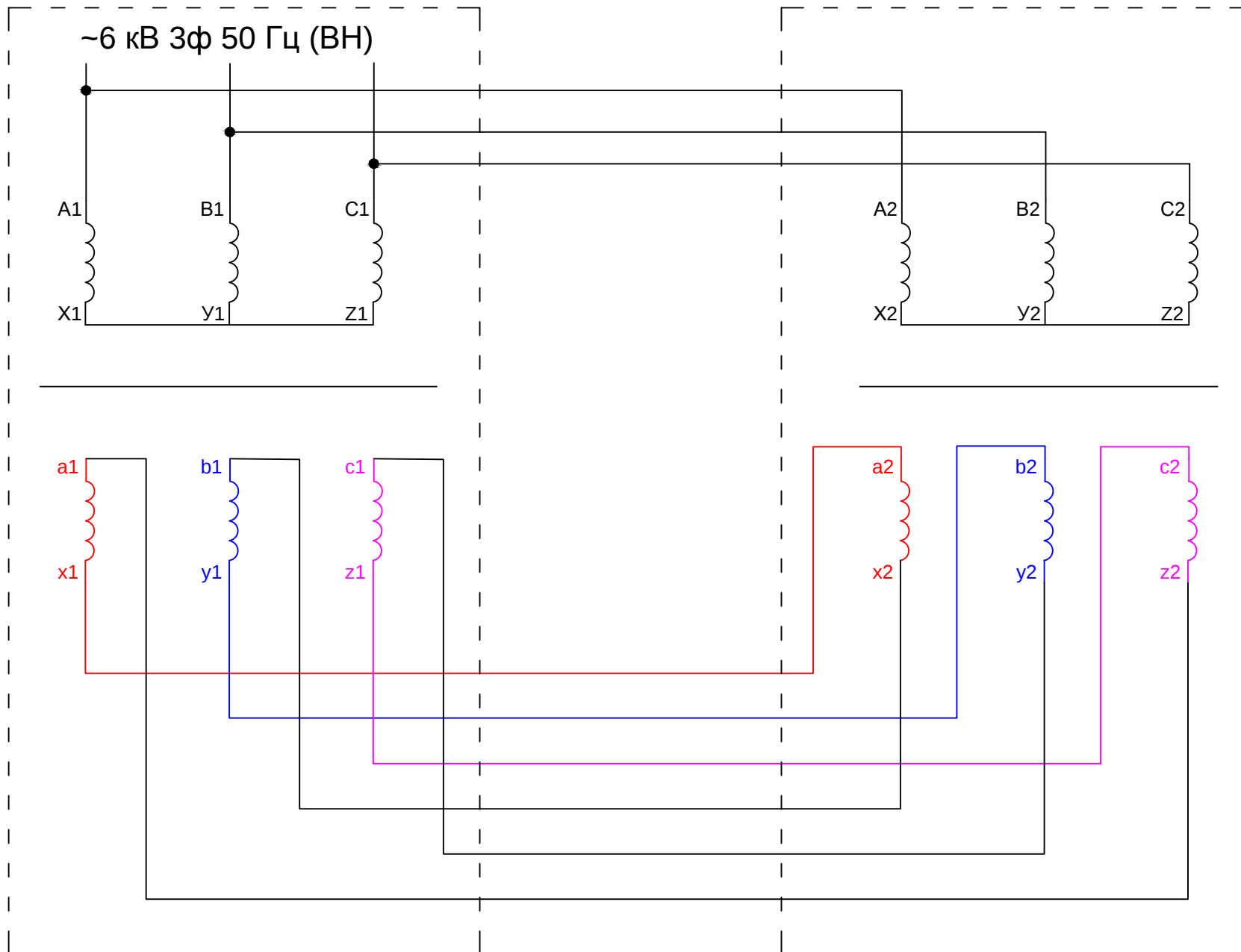
T1. TC3П 1000 кВа 6/0,4 кВ
