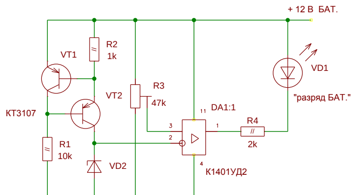
ОУ К1401УД2 как компаратор с однополярным питанием
