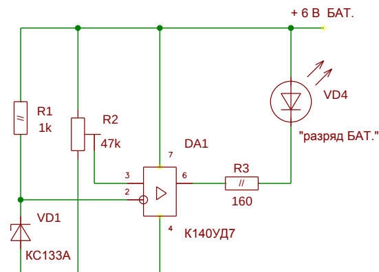
ОУ К140УД7 как компаратор с однополярным питанием
