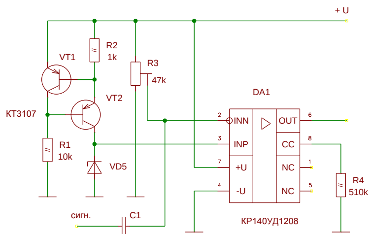
Программируемый ОУ КР140УД1208 как компаратор с однополярным питанием
