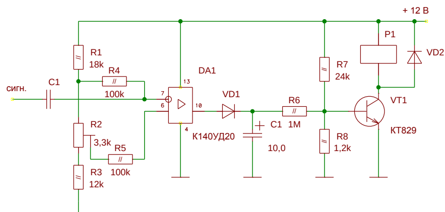
ОУ К140УД20 как компаратор с однополярным питанием
