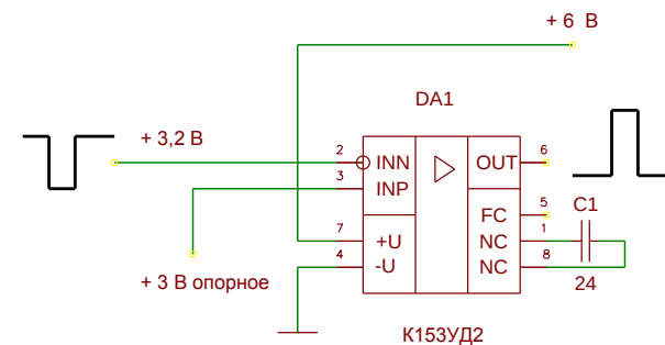
ОУ К153УД2 как компаратор с однополярным питанием
