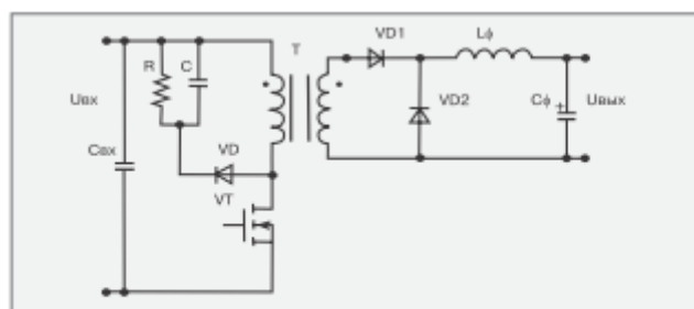
Рис. 32. Схема прямоходового преобразователя с RCD-демпфирующей цепочкой.
