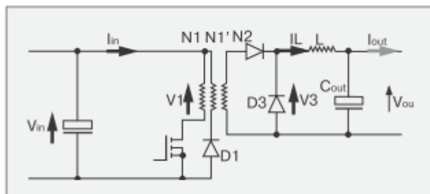
Рис. 13. Схема прямоходового [Forward] преобразователя.
