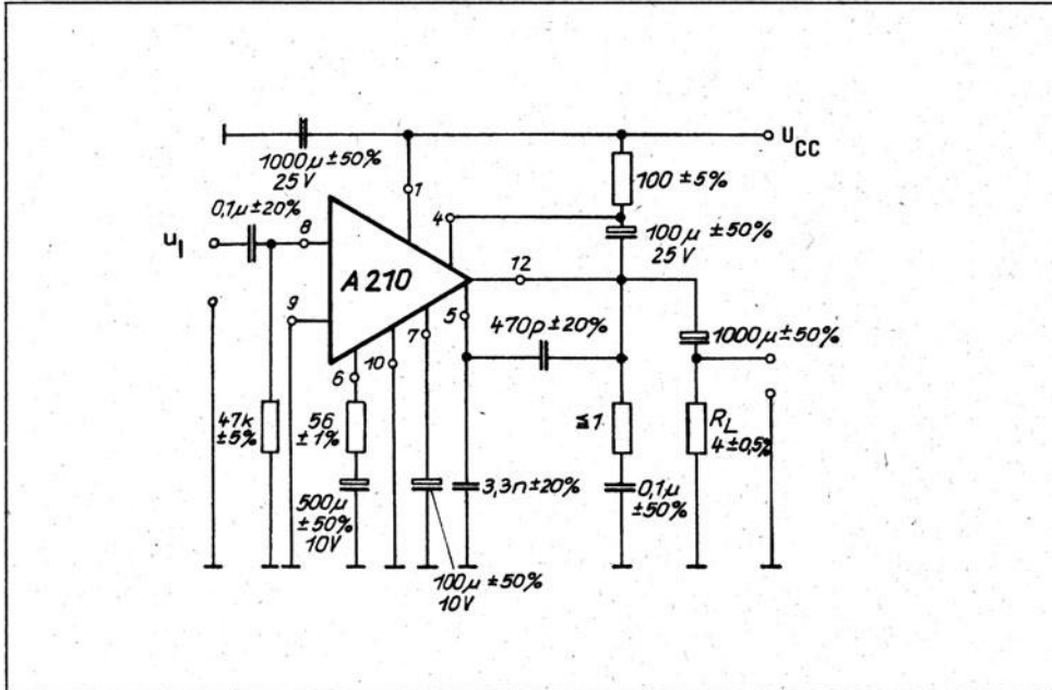
Meßschaltung
