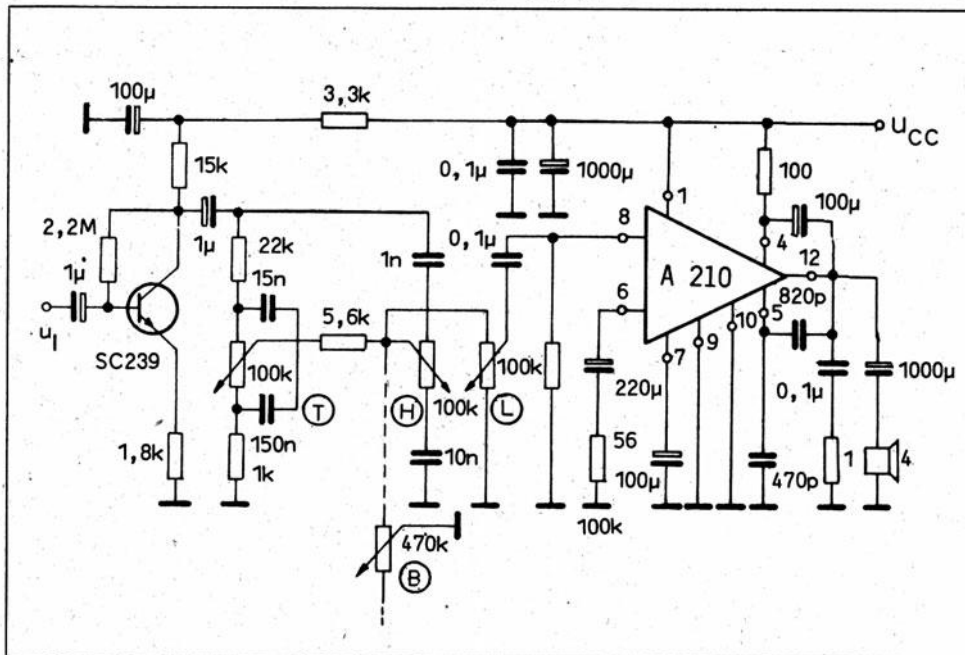
Applikationsbeispiel: NF-Verstärker für piezoelektrische Tonabnehmer /7/
