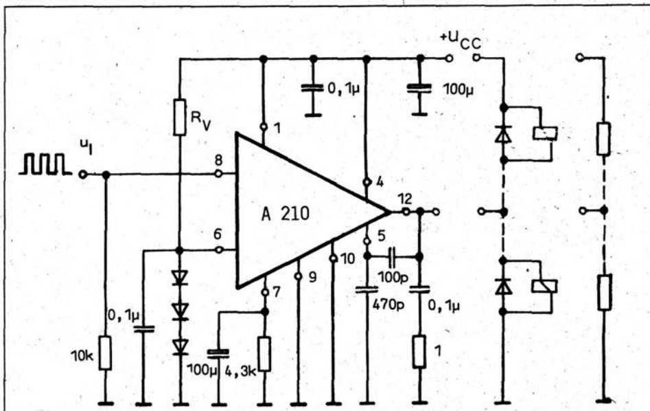
Applikationsbeispiel: Digitaler Schaltverstärker
