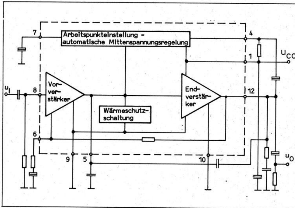
Übersichtsschaltplan
