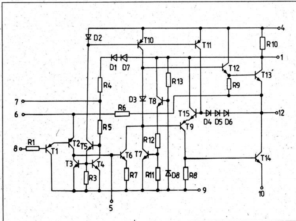
Innenschaltung
