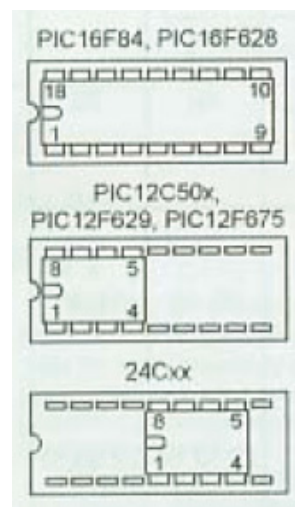
Установка различных микроконтроллеров в панель
