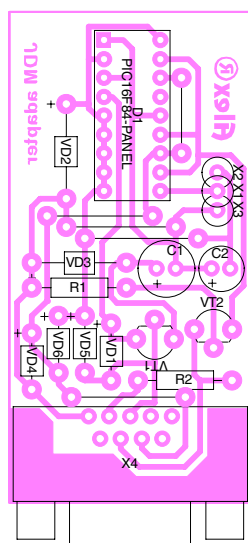
Компоновка элементов
