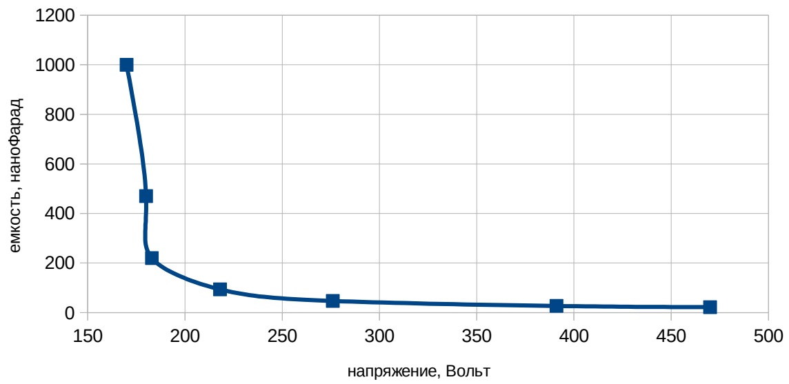
Зависимость напряжения на T2 от емкости C5
