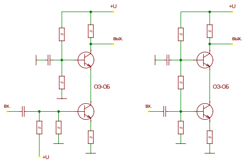
Каскоды ОЗ-ОБ с последовательным питанием
