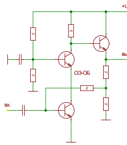
Каскод ОЗ-ОБ с последовательным питанием и автосмещением.
