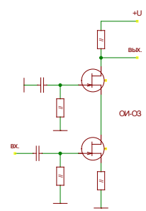
Каскод ОИ-ОЗ с последовательным питанием
