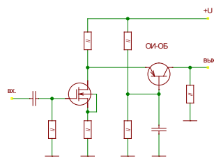
Каскоды с параллельным питанием
