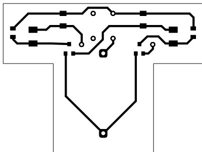
Верхний - зеркало
