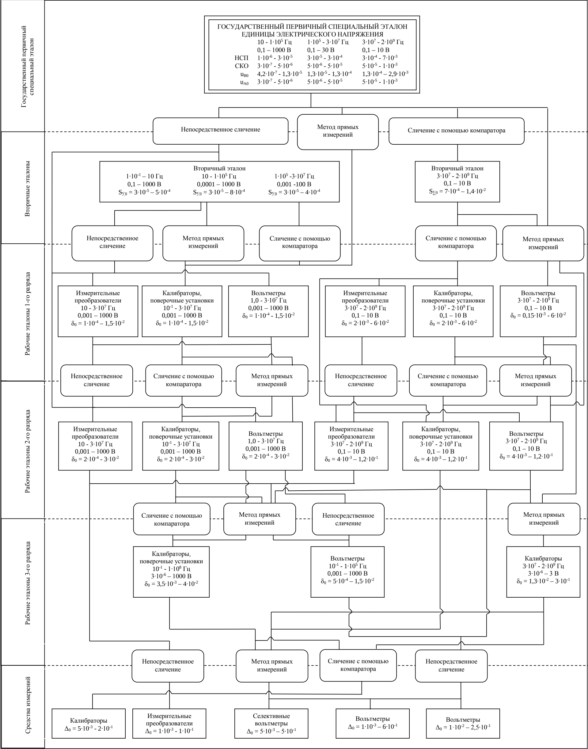
Государственная поверочная схема для средств измерений переменного электрического напряжения до 1000 В в диапазоне частот от 1 \cdot 10^{-1} до 2 \cdot 10^9 Гц
