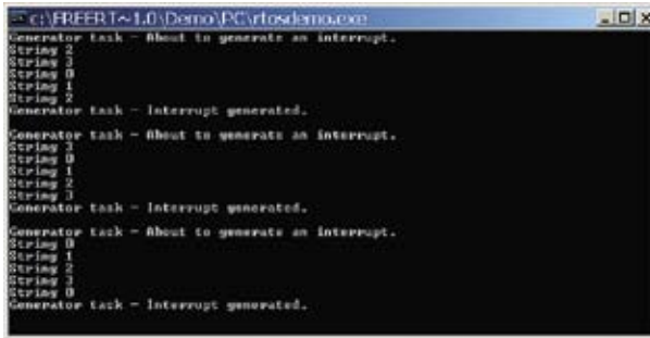
Рис. 11. Результаты выполнения учебной программы № 2
