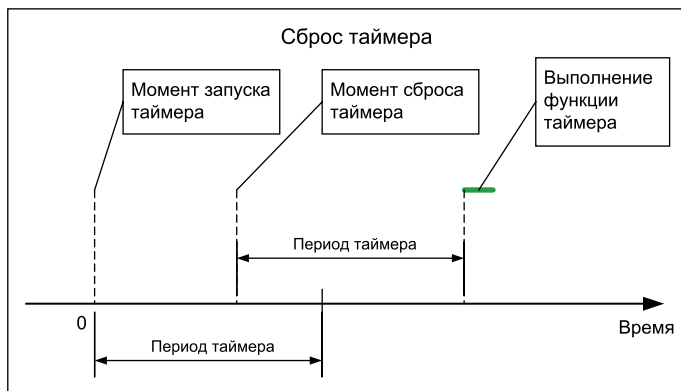
Рис. 3. Влияние сброса таймера на отсчет времени
