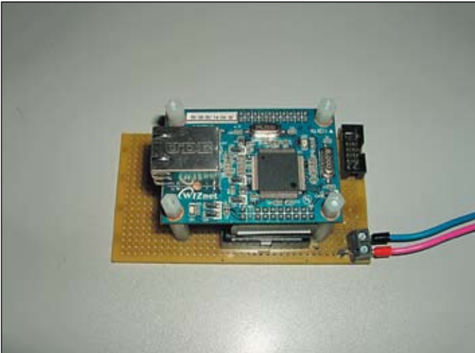
Рис. 6. Мезонинный модуль WIZ200WEB
