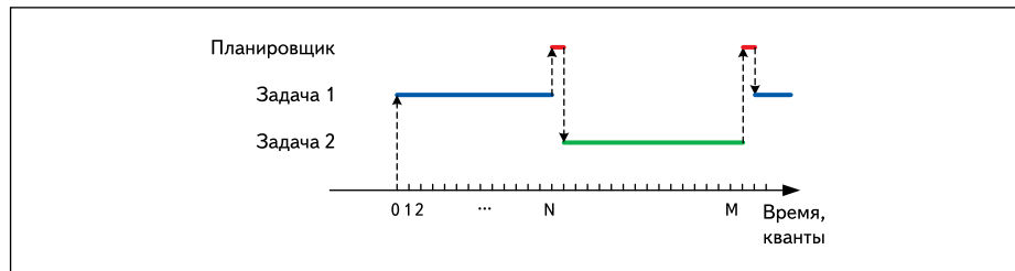
Рис. 7. Разделение процессорного времени между задачами при кооперативной многозадачности при явном вызове taskYIELD()
