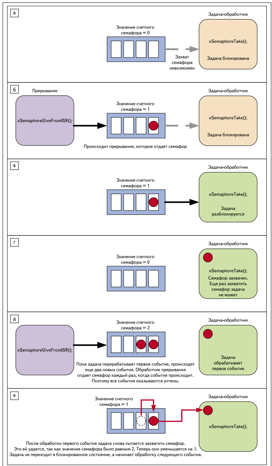
Рис. 8. Подсчет событий с помощью счетного семафора
