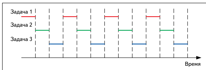
Рис. 2. Распределение процессорного времени между несколькими задачами в ОСРВ
