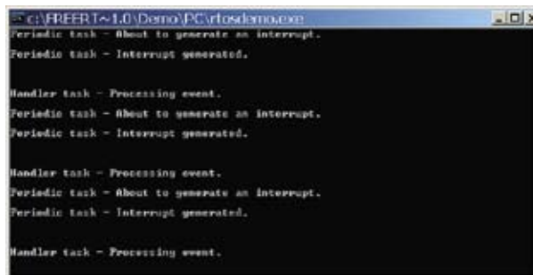
Рис. 6. Результаты выполнения учебной программы № 1 при отсутствии принудительного переключения контекста
