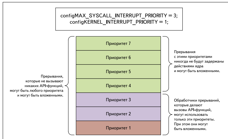
Рис. 13. Возможность вызова API-функций в обработчиках прерываний
