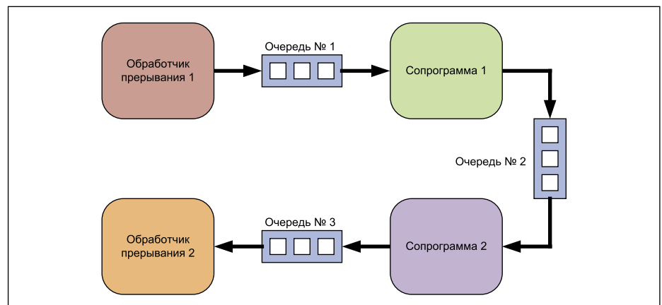
Рис. 5. Обмен сообщениями между сопрограммами и обработчиками прерываний в учебной программе № 2
