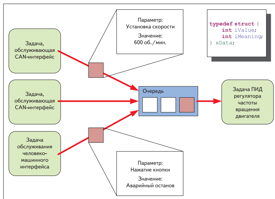
Рис. 5. Пример организации обмена информацией между задачами
