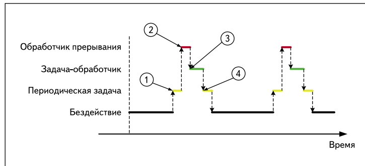
Рис. 5. Последовательность выполнения задач в учебной программе № 1
