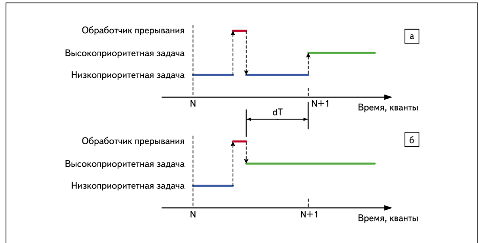
Рис. 3. Результат вызова xSemaphoreGiveFromISR() :
