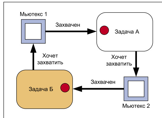
Рис. 8. Взаимная блокировка двух задач
