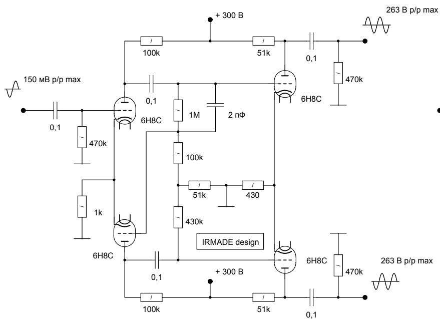
американский самобаланс 1938 года
