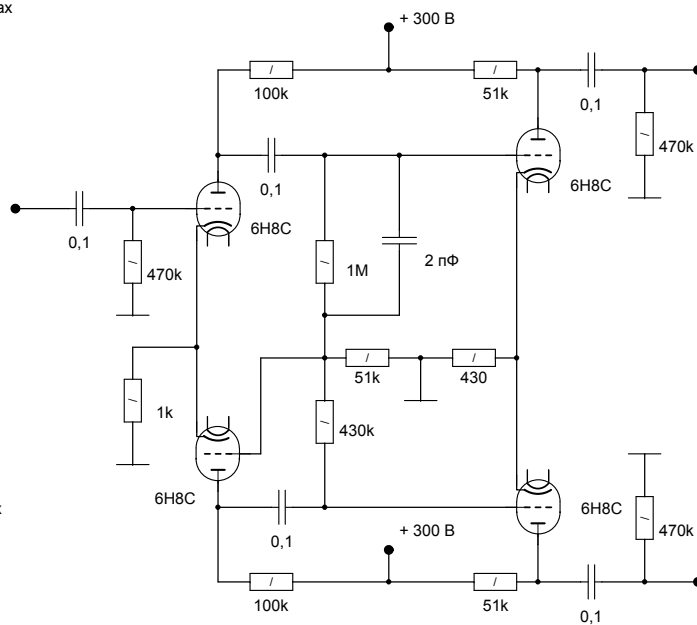
упрощённый самобаланс 1938 года, обладающий теми же свойствами.
