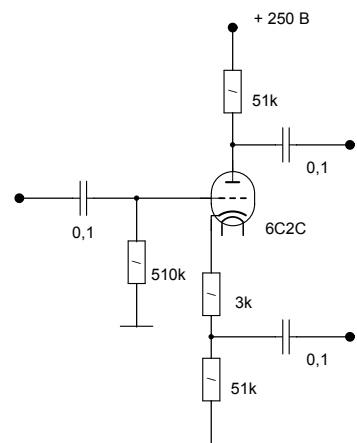
Парафазный каскад с разделённой нагрузкой по ср. с самобалансом имеет лучшую АЧХ.
