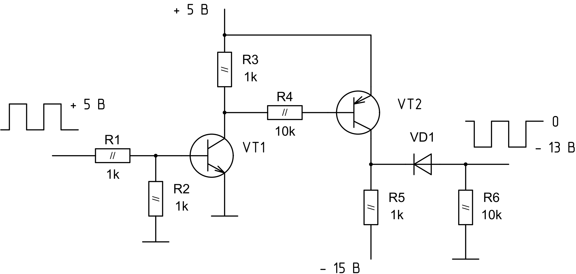
Преобразователь полярности импульсов
