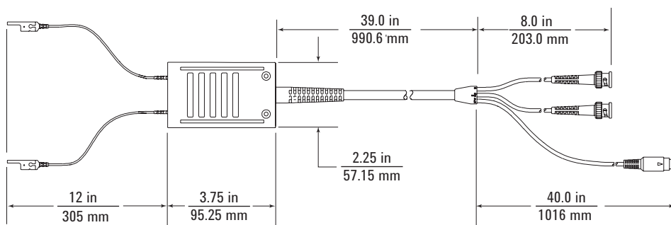
1145A dimensions
