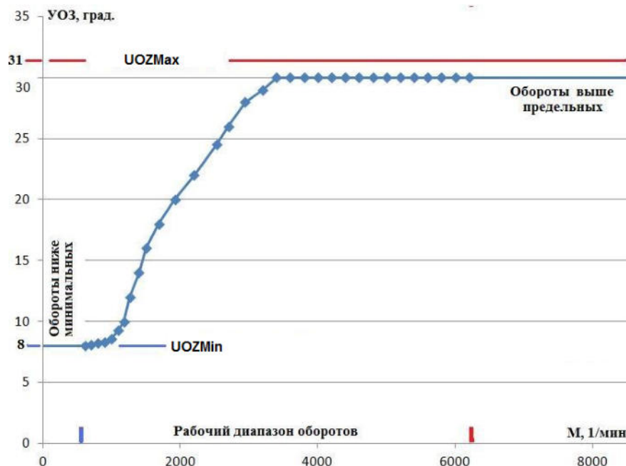
Рис. 11 Модельная зависимость УОЗ от оборотов
