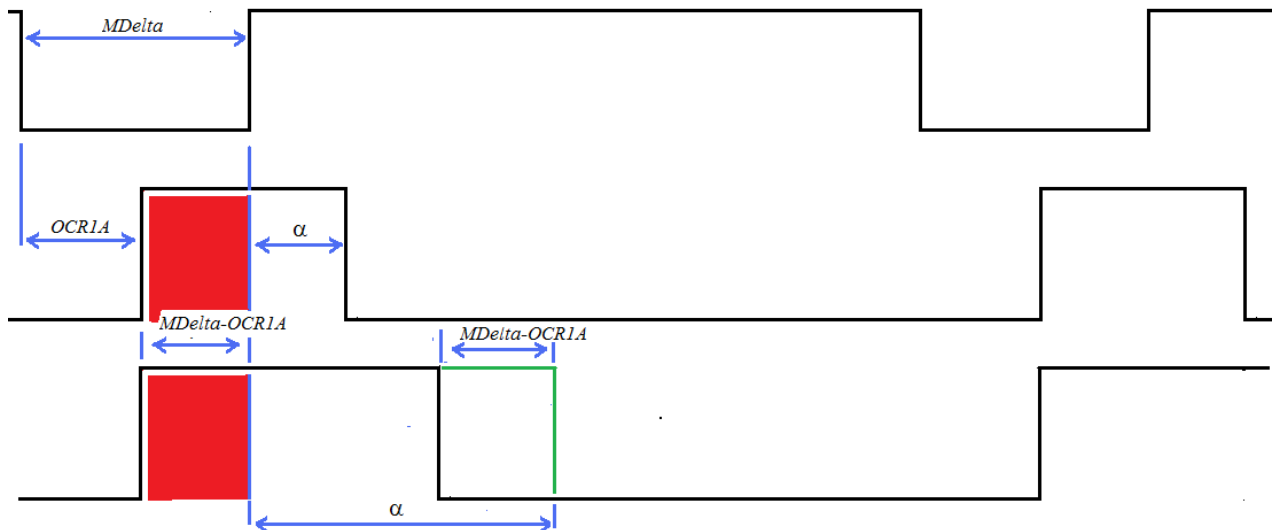
Рис. 8 Сигналы управления зажиганием и выходные каскады
