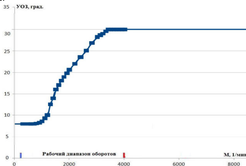
Рис. 12 Снижение нижнего уровня контролируемых оборотов.
