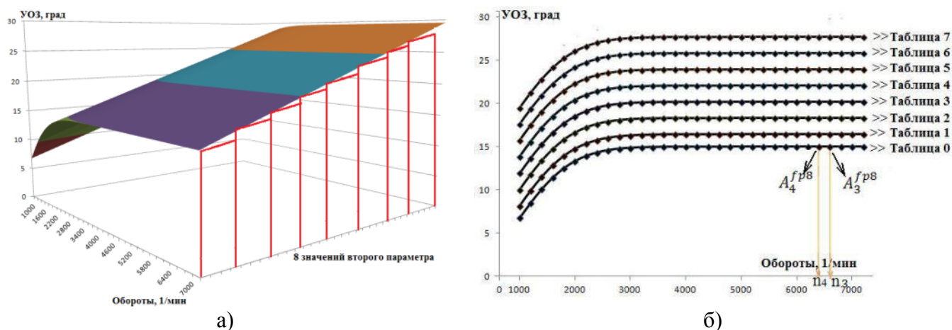
Рис. 7 Переход от аналитической зависимости \alpha(M, \dots) к таблицам A^{fp8}
