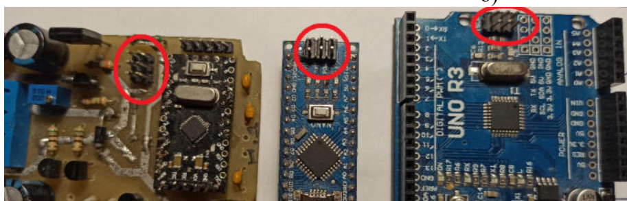
Рис. 15 Применение внутрисхемного программатора
