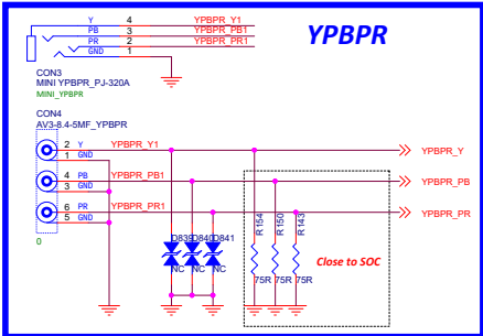
AV-IN1
