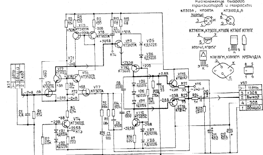
Усилителя корректирующего А1, А2
