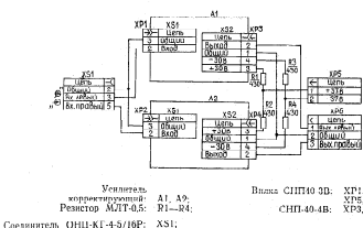
Усилителя корректирующего А1, А2
