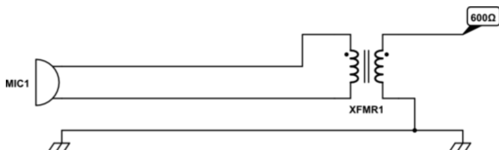
Рисунок 1. Использование трансформатора 1:1 для "разбалансировки" балансного микрофона для небалансного входа при сохранении балансной работы по всей длине кабеля.
