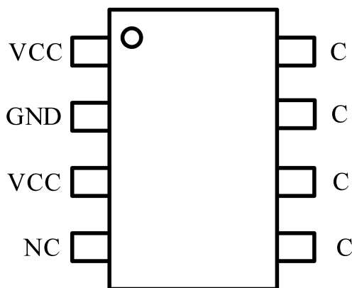
图 2 管脚封装图
