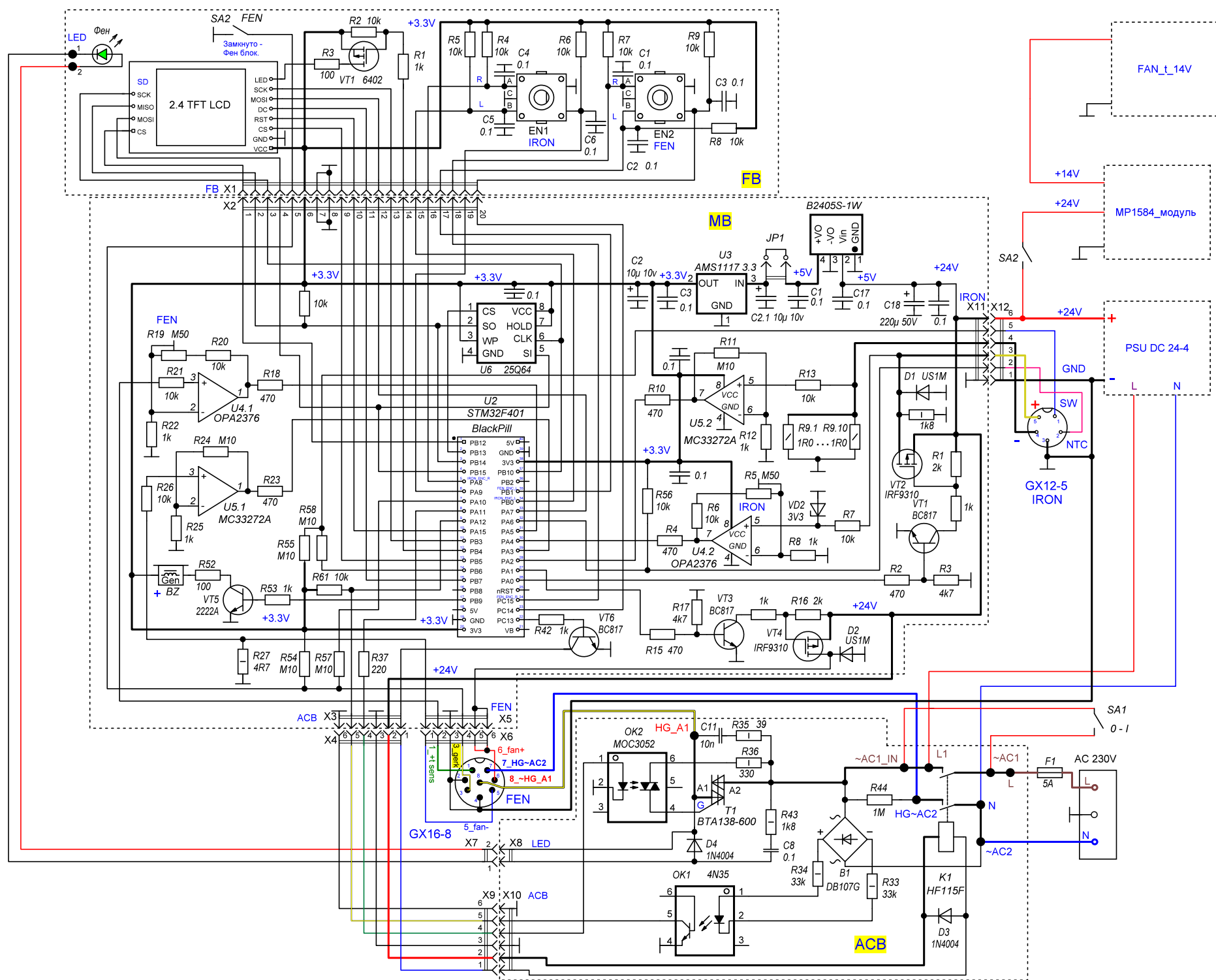
Схема станции
