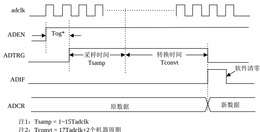
图 5-15 ADC 时序特征示意图
