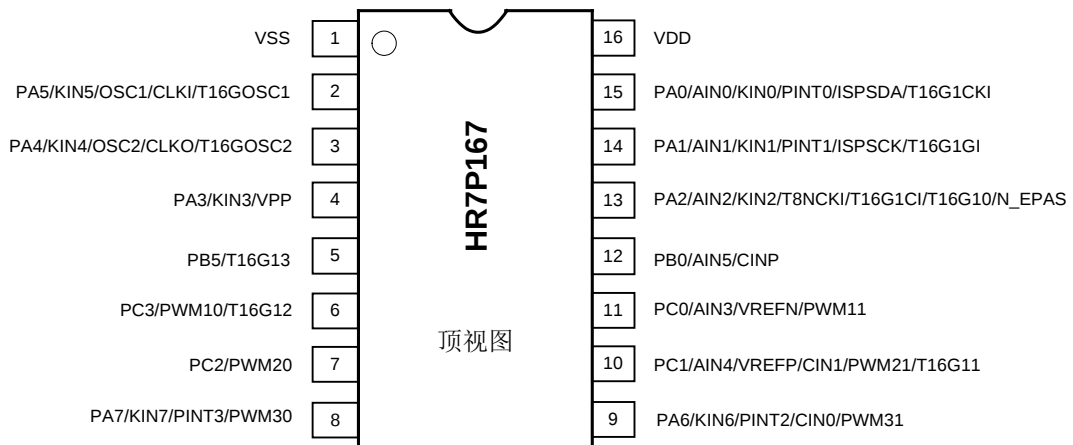
图 1-3 DIP16/SOP16 顶视图
