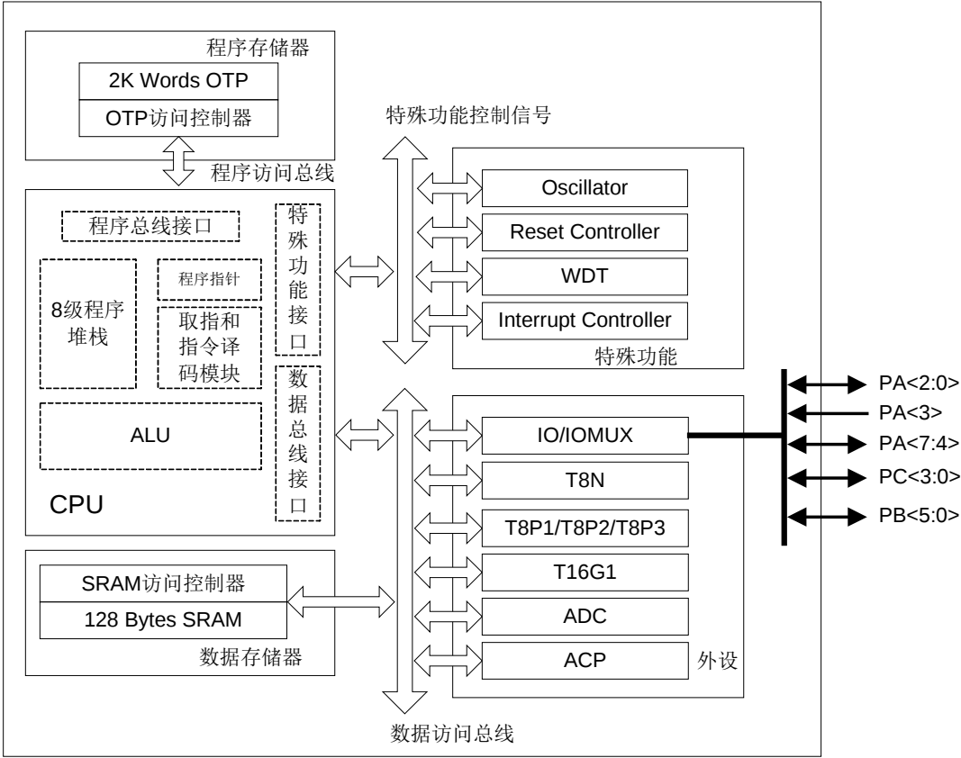
图 1-1 HR7P167 结构框图
