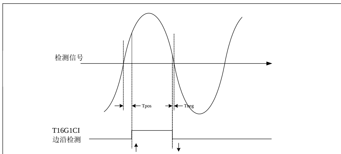
图 5-12 过零检测示意图
