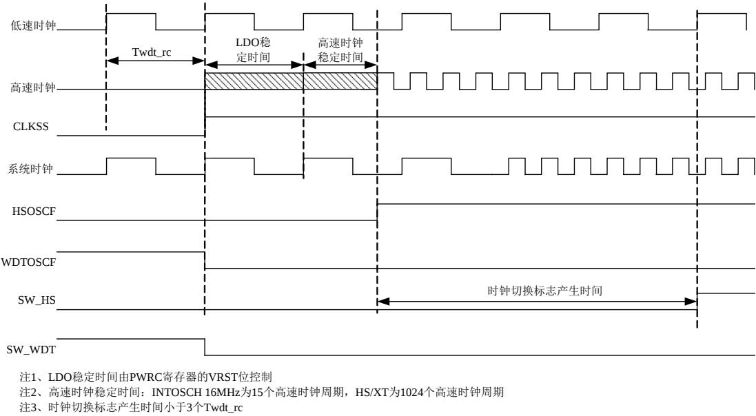
图 6-5 INTOSCL 时钟切换到 HS/XT/RC/INTOSCH 时钟时序图
