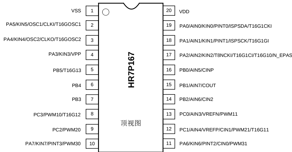
图 1-4 DIP20/SOP20/SSOP20 顶视图
