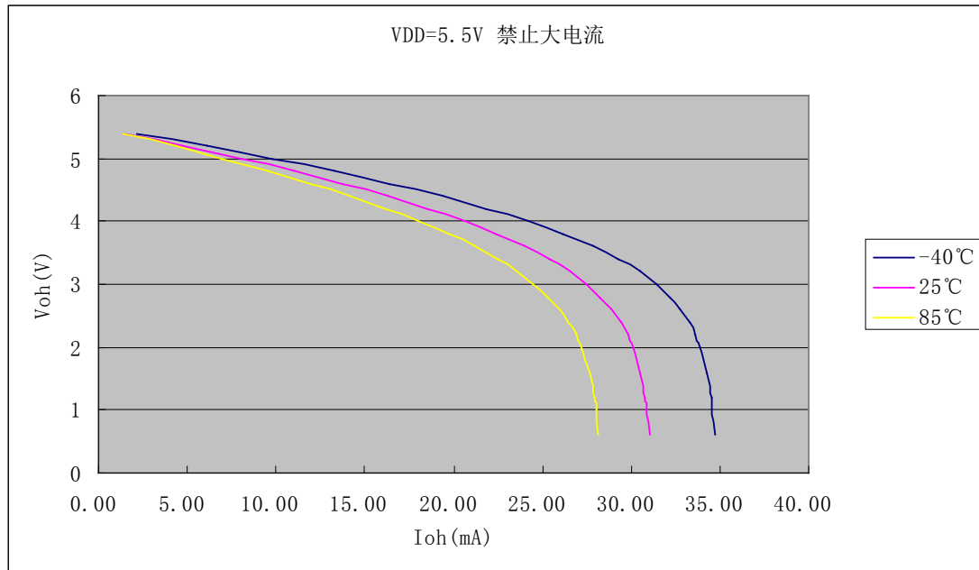
G: V_{OH} vs I_{OH} @VDD=5.5V
