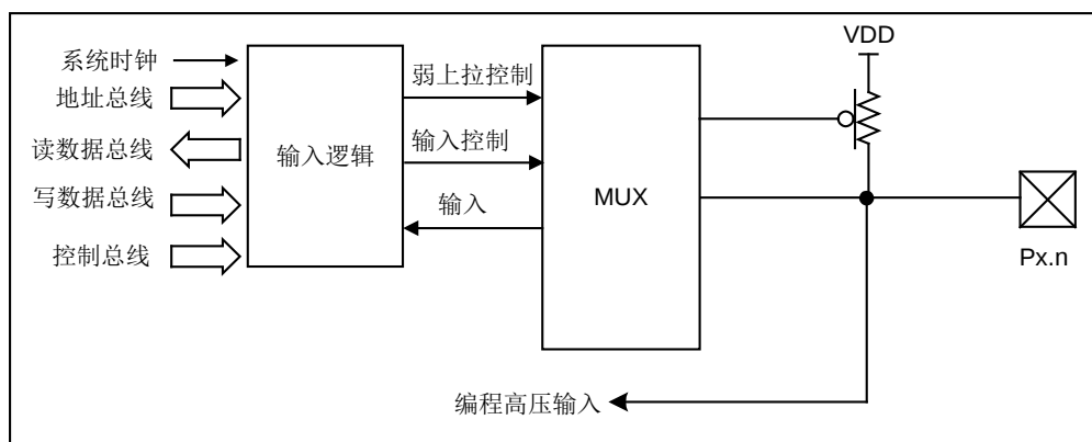
图 4-2 输入端口结构图 B
