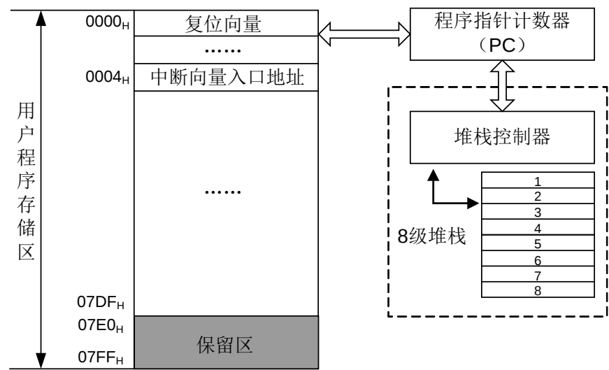
图 3-1 HR7P167 程序区地址映射和堆栈示意图
