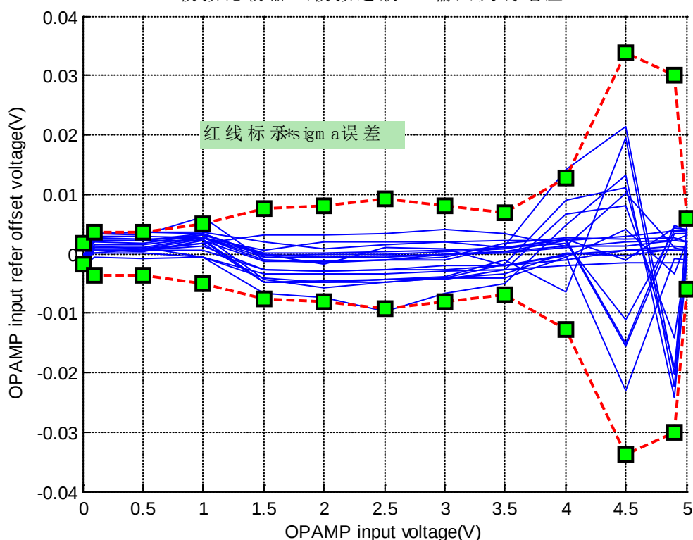
模拟比较器 ACP/模拟运放 OP 输入失调电压
