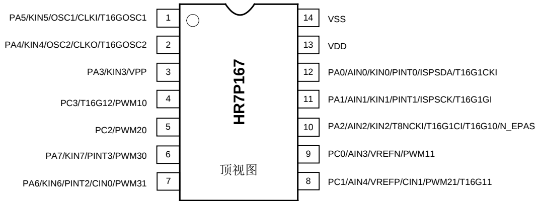
图 1-2 DIP14/SOP14 顶视图
