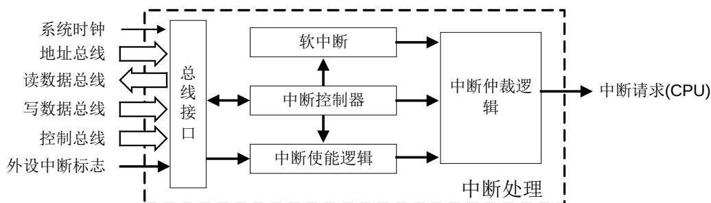
图 6-13 中断控制逻辑
