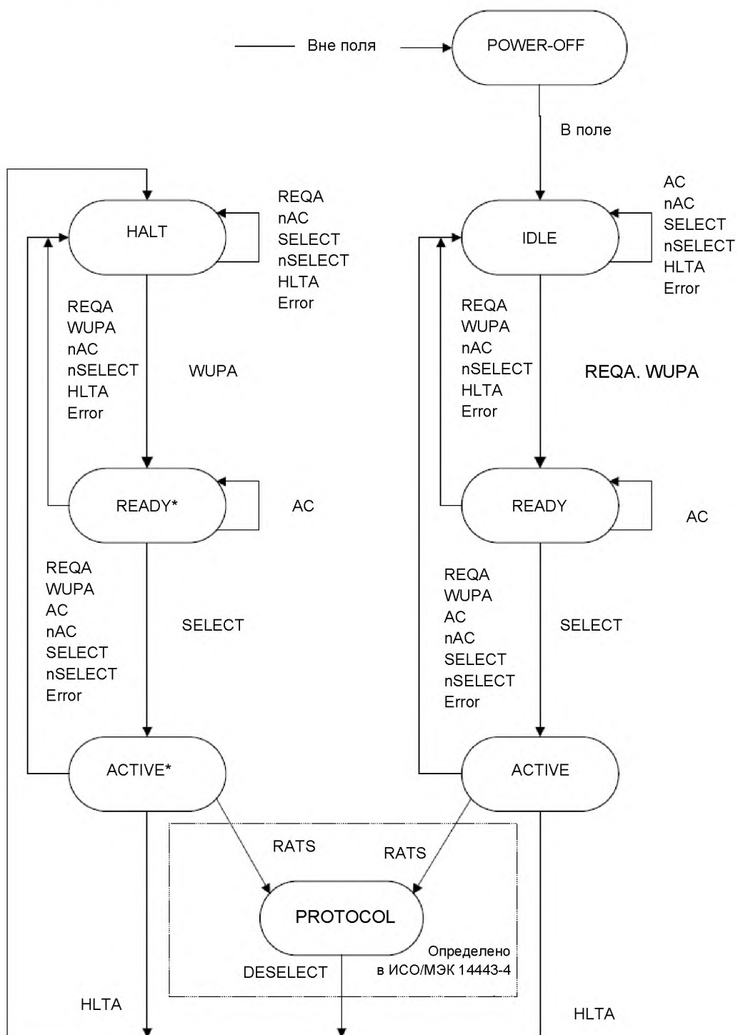
Рисунок 7 – Диаграмма состояний PICC типа А
