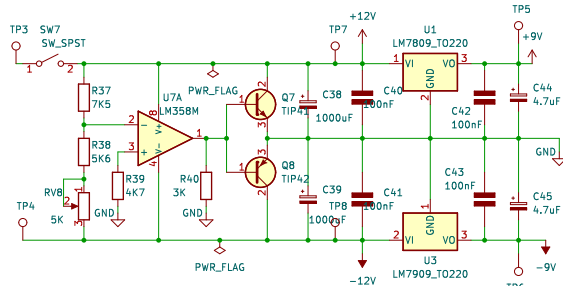
Двухполярное питание с однополярного источника питания LM358
