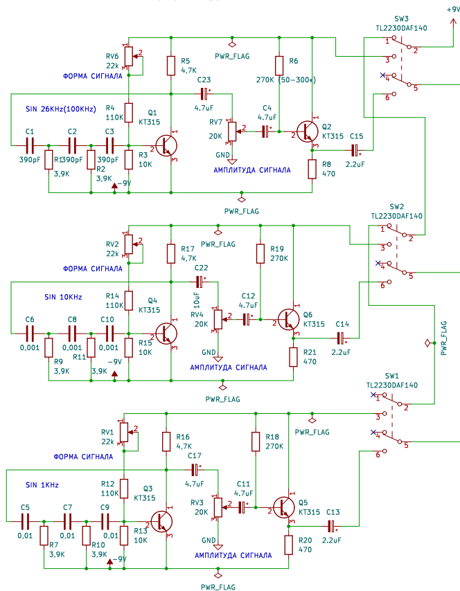
схема базового генератора для внутрисъемного диагностики
