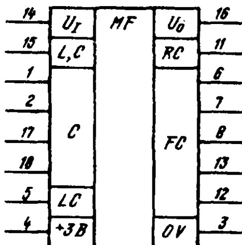
Условное графическое обозначение К174ХА34
