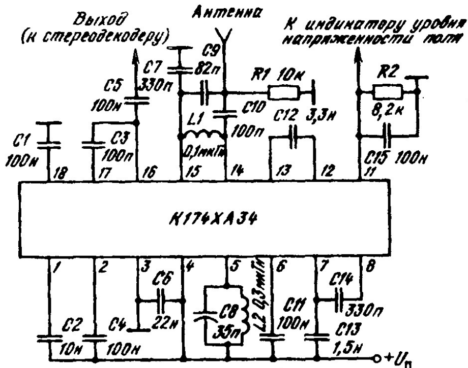
Типовая схема включения К174ХА34 в качестве стереофонического приемника. Значения элементов приведены для входного ЧМ сигнала с параметрами: f_{вх} = 69 МГц, \Delta f = \pm 50 кГц
