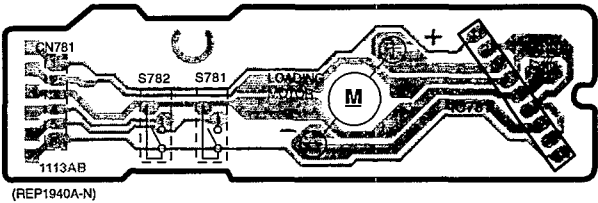
D LOADING MOTOR P.C.B.
