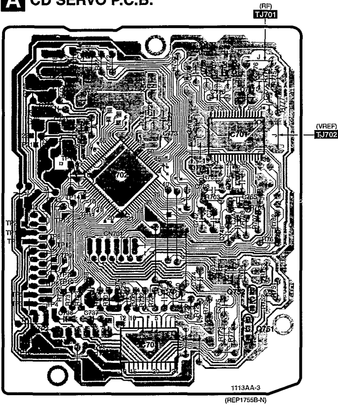
A CD SERVO P.C.B.
