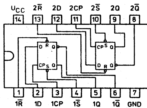
7474
