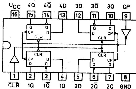
74175
