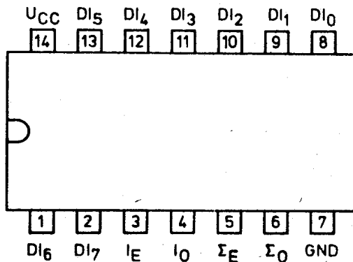
74180
