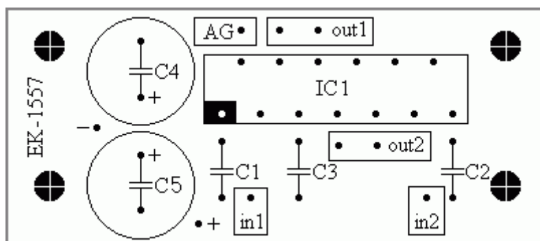
Расположение элементов на печатной плате
