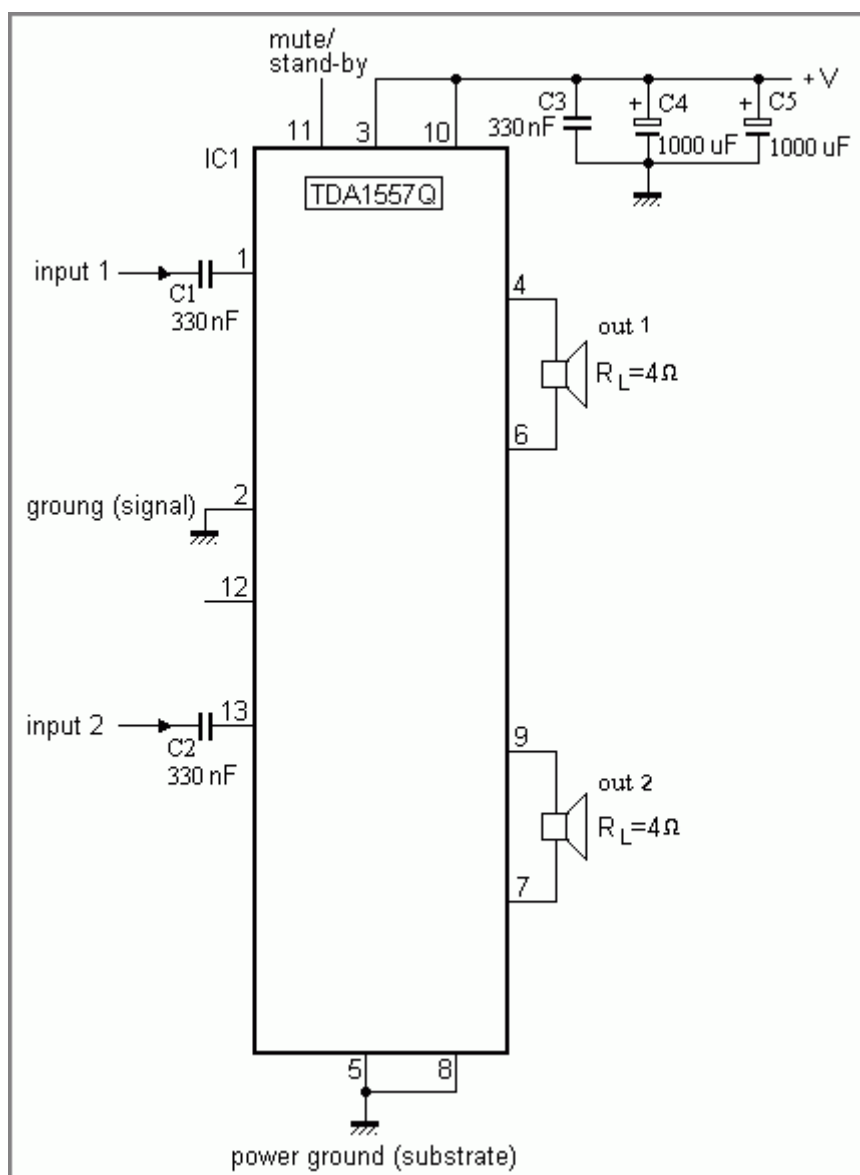
Схема электрическая принципиальная усилителя мощности
