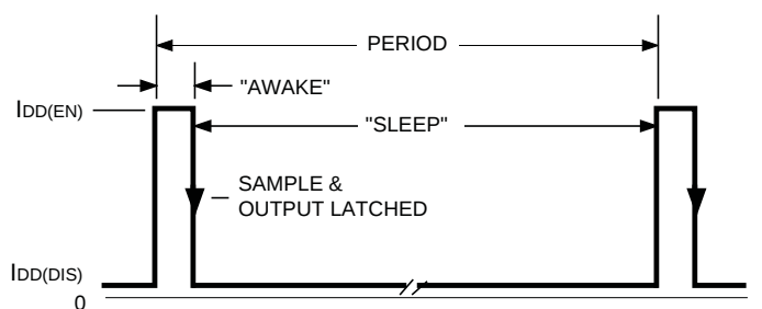
Dwg. WH-017-2
