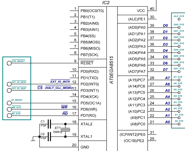
Адаптер-расширитель, режим аппаратно-программного УВБ. +5V
