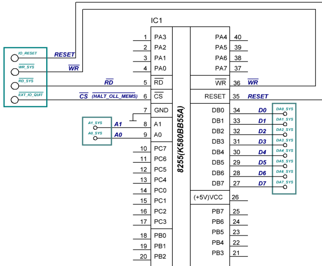
Адаптер-расширитель, классический УВБ
