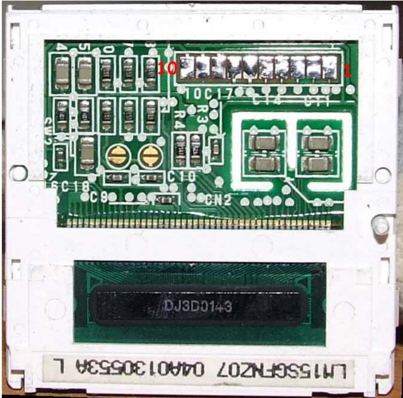
Siemens M55 LCD Module
